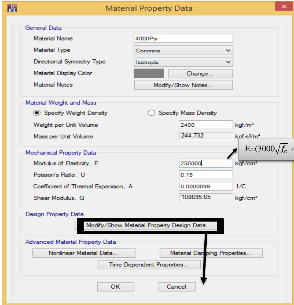
شکل ۸: تعریف مشخصات مصالح بتنی
