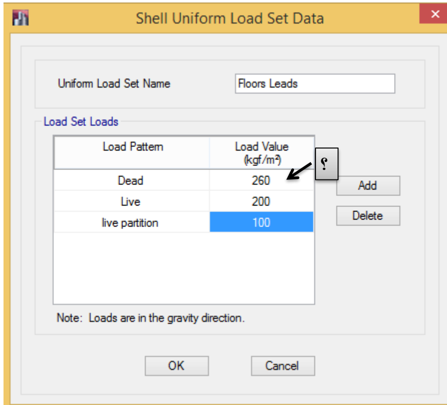
شکل ۷۷: بسته بارگذاری گسترده طبقات
