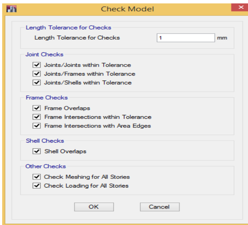
شکل ۸۷: کنترل مدلسازی
