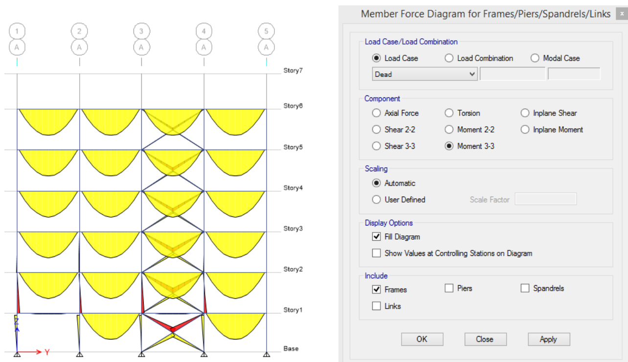
شکل ۹۱: نمایش نیروهای داخلی المانها
