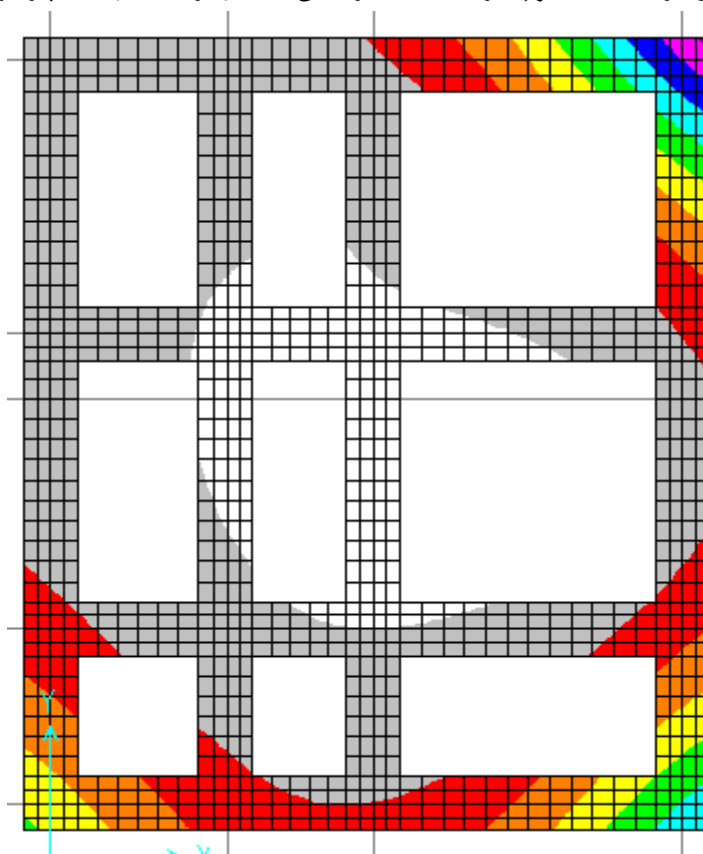
تنش‌های موجود در زیر پی نشان داده شده در نرم‌افزار
